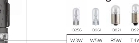
W3W W5W R5W T4W
