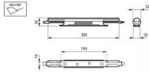
BCX422 2700 HE L305 CE/CCC Dimensions en mm.
