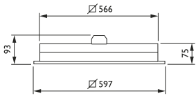
RC360BW60L60 Dimensions en mm
