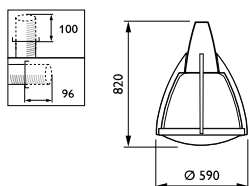
CDS590/592/594 Dimensions en mm.
