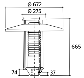
Osiris BDS770 (FSD-36). Dimensions en mm.
