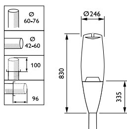
CDS530/531 Dimensions en mm.
