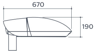
Arc LED 80 (BGP618) Verre plat. Dimensions en mm.
