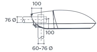
Détails de montage. Dimensions en mm.
