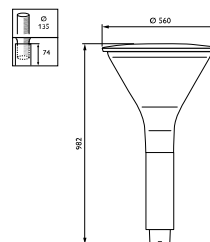
BDS670 Dimensions en mm.
