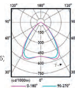
SM134V OC, BAP-tauglich
