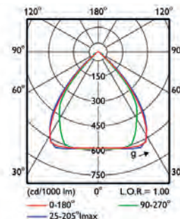
BY471P MB, tief-/breitstrahlend
