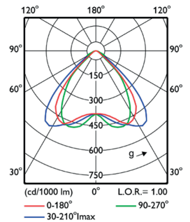
BY471P WB, breitstrahlend
