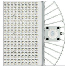
In der neuen PIR-Version wird die Leuchte mit integriertem Bewegungssensor geliefert. Die fest voreingestellte Steuerung schaltet automatisch nach 15 min ohne Bewegung auf 25% des Lichtstromes. Damit sind zusätzlich deutliche Kosteneinsparungen möglich.
