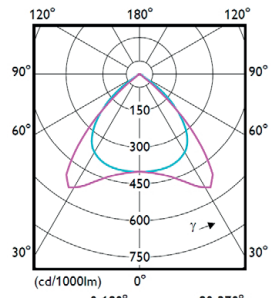
Breitstrahlende Optik (WB)
