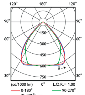
BY471P MB, tief-/breitstrahlend
