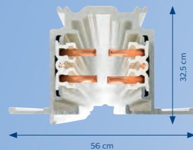
Einbauvariante
