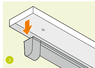
3 Open the 4ft batten. Disconnect gear inside (no need for gear for TLED) 打开 4 英尺灯具 断开内部的镇流器 (TLED 不需要镇流器)
