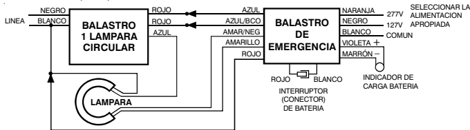
K) CON BALASTRO NORMAL PARA DOS (2) LAMPARAS DE ENCENDIDO INSTANTANEO EN CIRCUITO SEQUENCIA SERIE. DESDE 17 W HASTA 40 W TUBO T8, T10, o T12.
