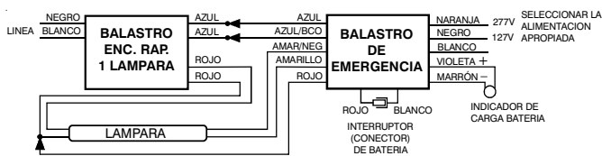
A) CON BALASTRO NORMAL PARA UNA (1) LAMPARA DE ENCENDIDO RAPIDO DESDE 17W HASTA 215W.
