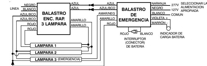
I) CON BALASTRO NORMAL PARA TRES (3) LAMP DE BALASTRO ELECTRONICO.
