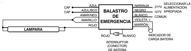
M) SIN BALASTRO NORMAL. PARA INSTALARSE SOLAMENTE CON UNA LAMPARA FLUORESCENTE DESDE 17W HASTA 40W TUBO T8, T10, o T12.
