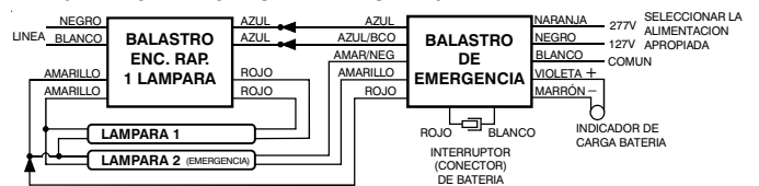
B) CON BALASTRO NORMAL PARA DOS (2) LAMPARAS DE ENCENDIDO RAPIDO DESDE 17W HASTA 215W.
