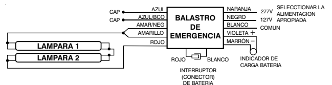
N) SIN BALASTRO NORMAL. PARA INSTALARSE CON DOS (2) LAMPARAS FLUORESCENTES DESDE 17W HASTA 40W TUBO T8, T10, o T12.
