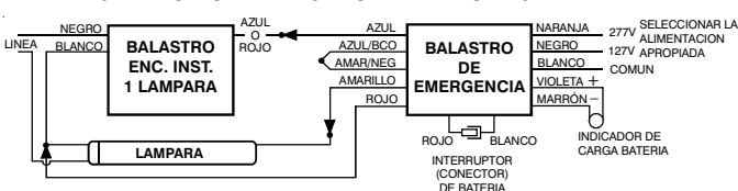
C) CON BALASTRO NORMAL PARA UNA (1) LAMPARA DE ENCENDIDO INSTANTANEO DESDE 17W HASTA 75W.
