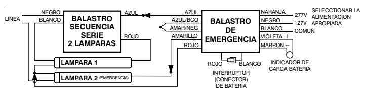
D) CON BALASTRO NORMAL PARA DOS (2) LAMPARAS DE ENCENDIDO INSTANTANEO EN CIRCUITO SECUENCIA SERIE. DESDE 17W HASTA 75W.
