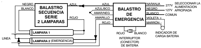
E) CON BALASTRO NORMAL PARA DOS (2) LAMPARAS DE ENCENDIDO INSTANTANEO EN CIRCUITO SEQUENCIA SERIE. DESDE 17W HASTA 75W.
