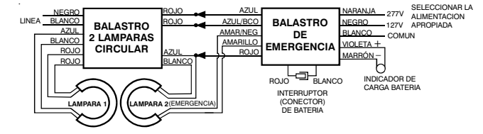
H) CON BALASTRO NORMAL PARA DOS (2) LAMPARAS CIRCULARES DE ENCENDIDO RAPIDO.
