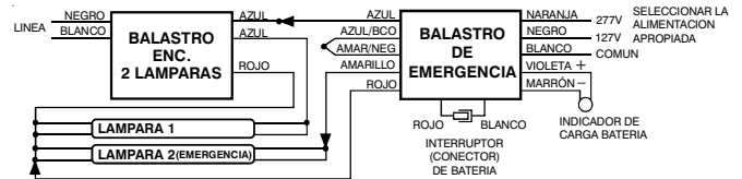
F) CON BALASTRO NORMAL PARA DOS (2) LAMPARAS DE BALASTRO ELECTRONICO.
