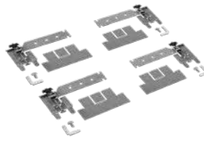
ZBS460 SMB Montagebeugelset voor bevestiging in systeemplafonds met verdekte profielen
