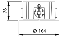
ZCP780 MB - Afmetingen in mm
