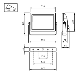
BCP414-415 MP - Afmetingen in mm.
