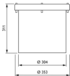
ZBP523 RMB-RND Afmetingen in mm.
