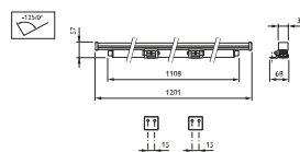
BCP421_422 L1200 Afmetingen in mm.
