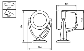
Afmetingen in mm.
