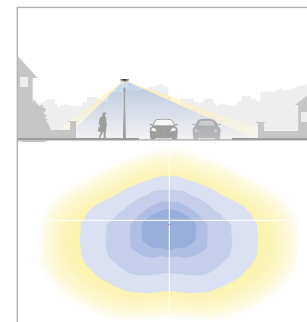
Vertikal ljusfördelning för gång- och cykelvägar
