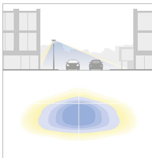
Mediumstrålände ljusfördelning för gatubelysning
