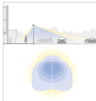
Asymmetrisk ljusfördelning för arealbelysning
