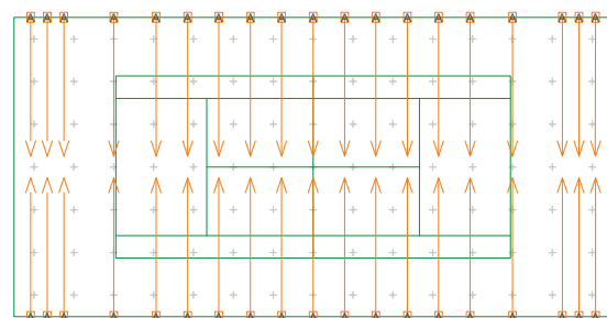
Strålkastarnas inriktning
