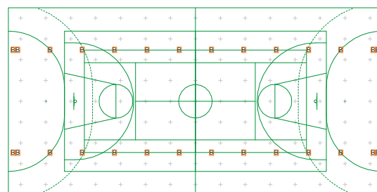
Strålkastarnas inriktning
