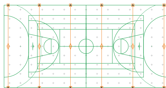
Strålkastarnas inriktning
