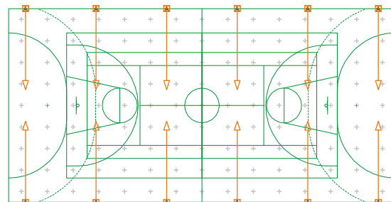
Strålkastarnas inriktning
