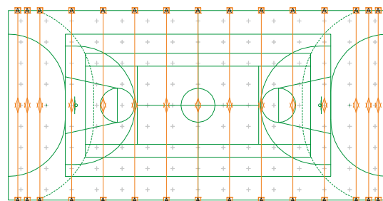
Strålkastarnas inriktning
