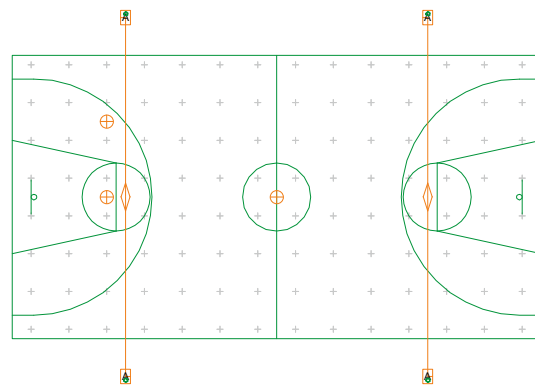
Strålkastarnas inriktning
