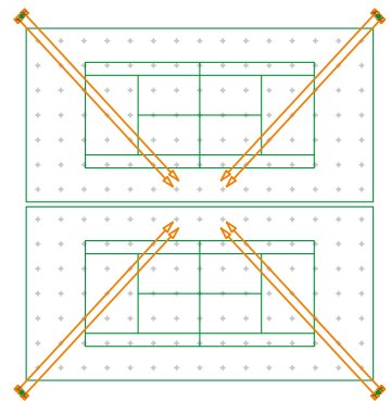
Strålkastarnas inriktning
