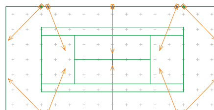
Strålkastarnas inriktning
