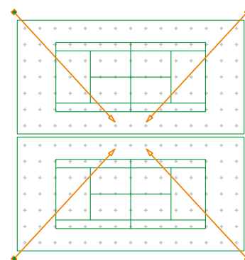
Strålkastarnas inriktning
