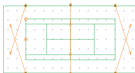
Strålkastarnas inriktning
