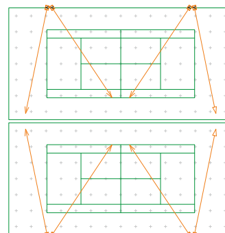
Strålkastarnas inriktning
