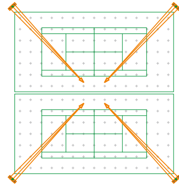
Strålkastarnas inriktning
