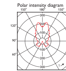
6-40W E14 2700K
