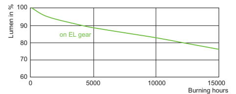
CDM-T Accent 35W /930
