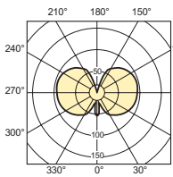
CDM-T Elite 35W /842, /930, /942
