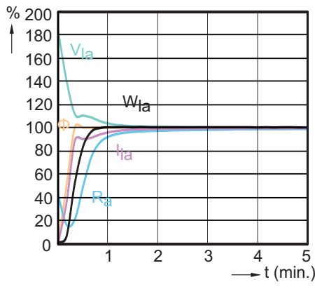
CDM-T Elite 50W /930
