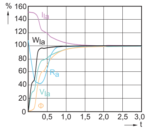
CDM-T Fresh 70W /740
