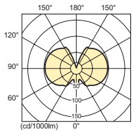
CDM-T Fresh 70W /740
