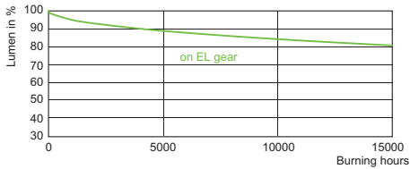
CDM-T Elite 35W /842, /942
