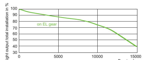
CDM-T Fresh 70W /740
