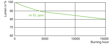
CDM-TC Accent 50W & 70W /930
