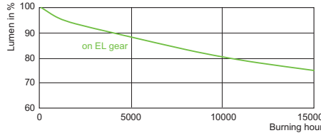
CDM-TC Accent 35W /930
