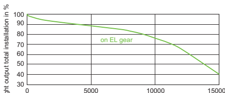
CDM-T Elite 50W, 70W /942
