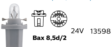
Base Plástica Cinza (BAX1,2W GREY)
