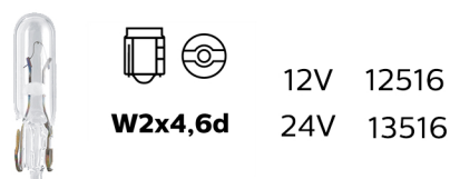
Pinguinho de 1W
