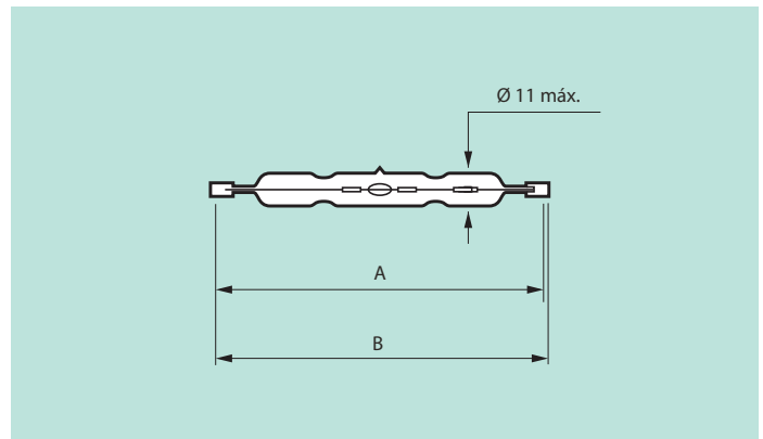
Diagramas de dimensiones en mm
