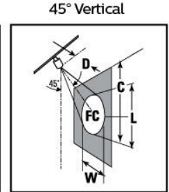
45° Ángulo de alineación vertical
