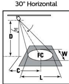
30° Ángulo de alineación horizontal
