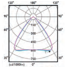
SM530C, BAP-tauglich
