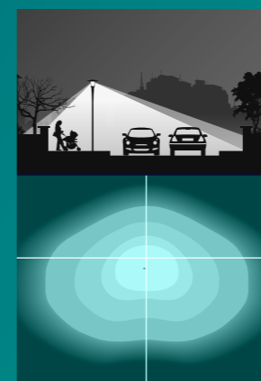
DV Lichtverdeling Breed voor verticale verlichtingssterkte
