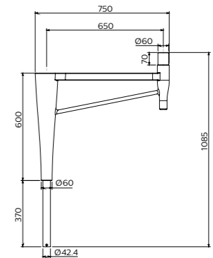
Eenarmige uithouder
