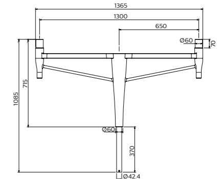
Tweearmige uithouder
