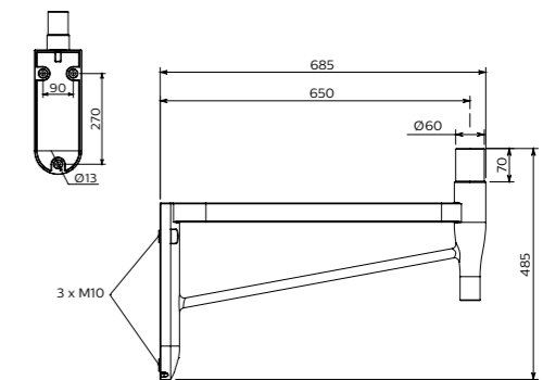
Wandmontage-uithouder
